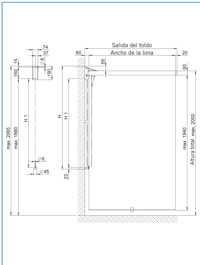
Ejemplo de fijación a pared
