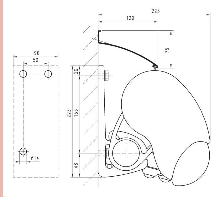
Ejemplo de fijación a pared con protector
