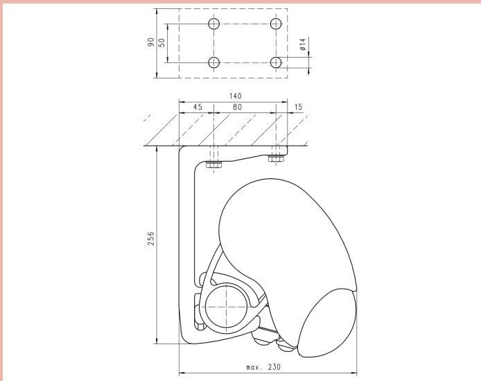
Ejemplo de fijación a techo
